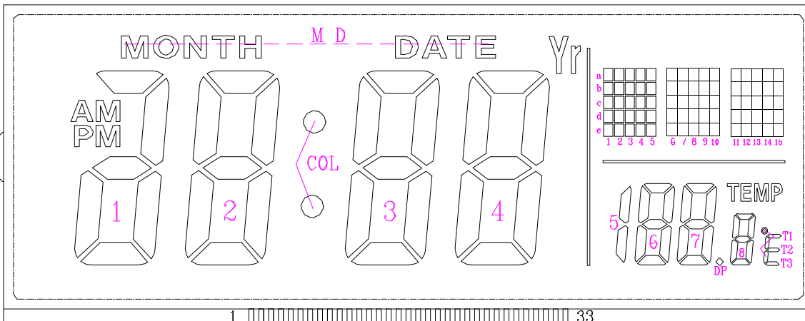
COM0~COM4,SEG0~SEG27
