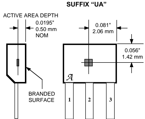
Dwg. MH-011-7A
