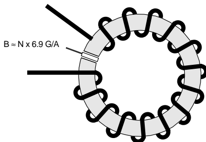
Dwg. AH-005A
