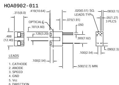
外形尺寸图, 单位为英寸 (毫米)
