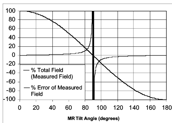
图6 - 满量程输出，与传感器的倾斜角
