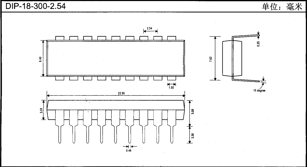
封装外形图
