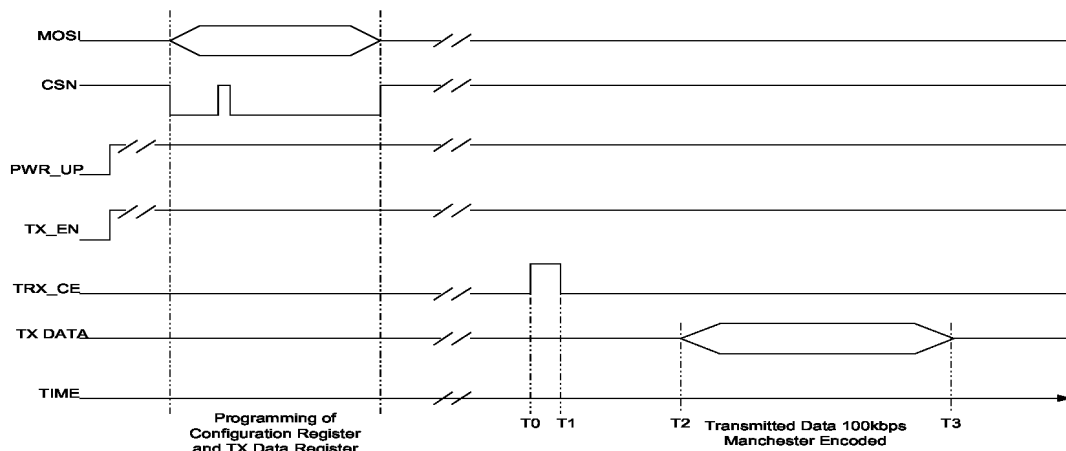
发射时序图
