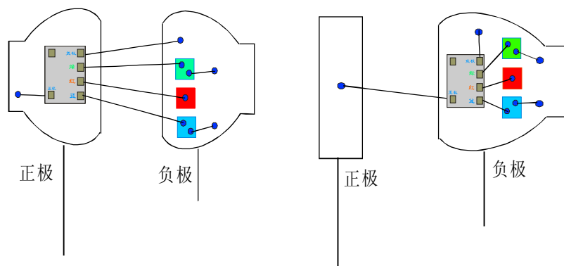
支架焊线图
