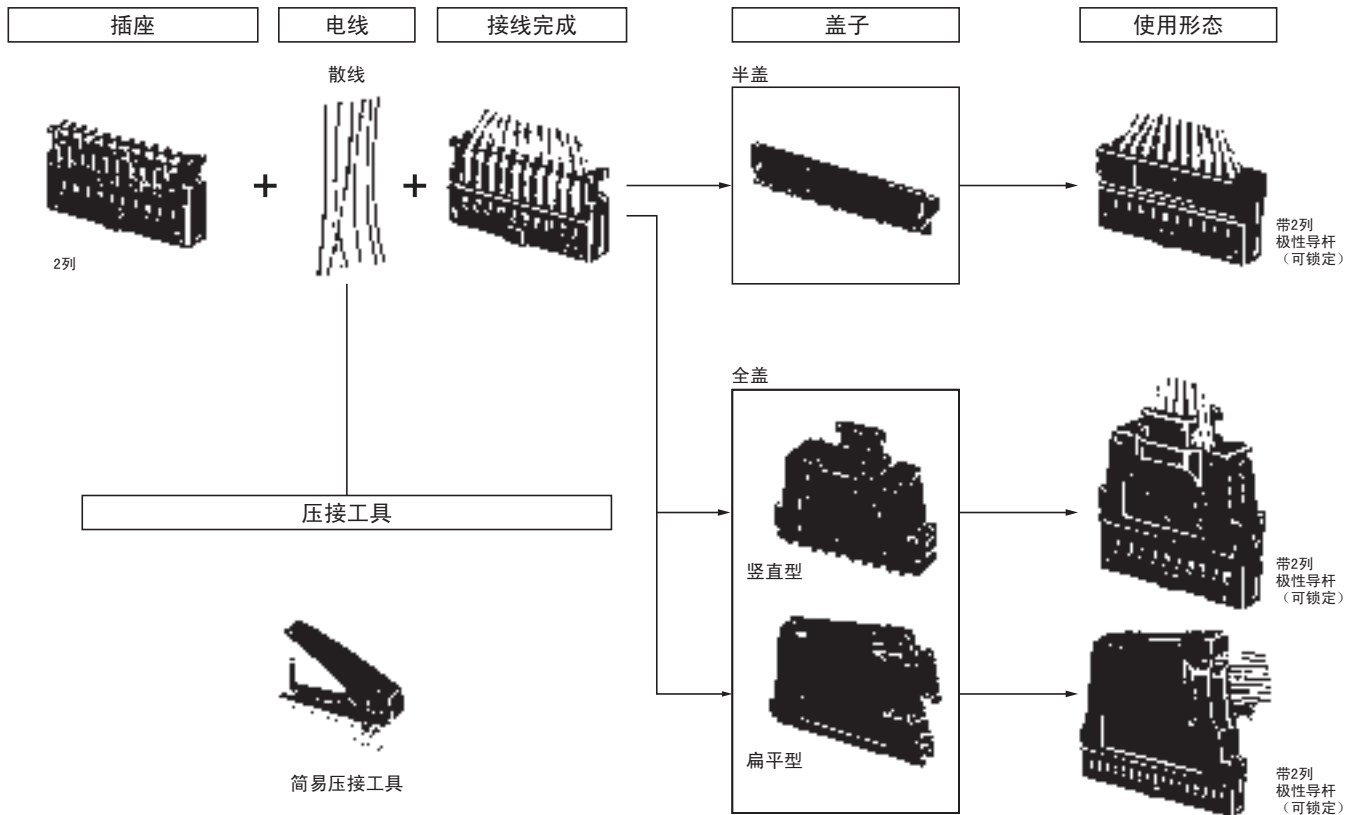
组装结构图
