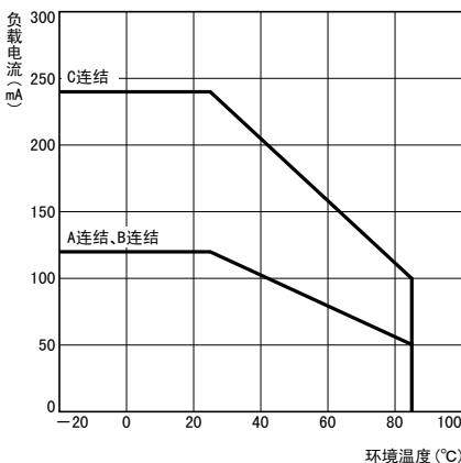
负载电流—环境温度 G3VM-353H
