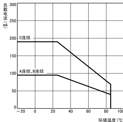
负载电流—环境温度 G3VM-353H1
