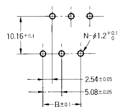
印刷基板加工尺寸 (BOTTOM VIEW) 适合基板厚度: 1.6mm
