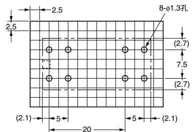
印刷基板加工尺寸 (BOTTOM VIEW) 尺寸公差为±0.1mm
