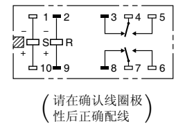
端子配置/内部连接图 (BOTTOM VIEW)
