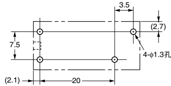
安装孔加工尺寸 (BOTTOM VIEW) 尺寸公差为±0.1mm
