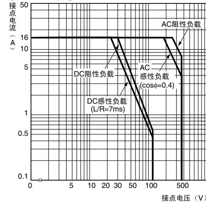
G2R-1-E、G2R-1A-E
