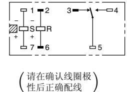
端子配置/内部连接图 (BOTTOM VIEW)
