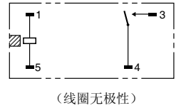
端子配置/内部连接图 (BOTTOM VIEW)
