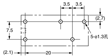
安装孔加工尺寸 (BOTTOM VIEW) 尺寸公差为±0.1mm
