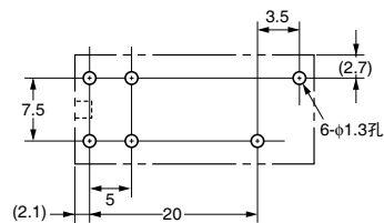
安装孔加工尺寸 (BOTTOM VIEW) 尺寸公差为±0.1mm
