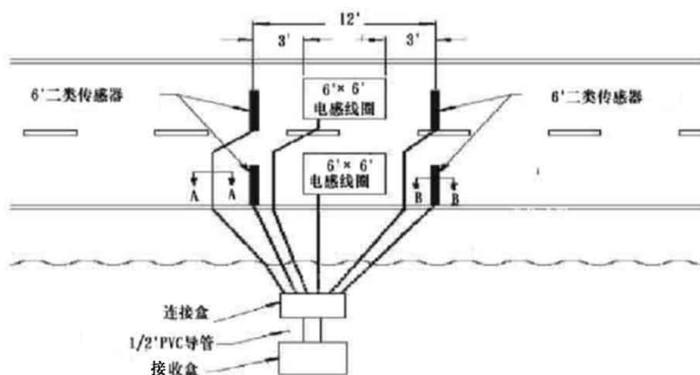
对 1.8 米二类传感器,典型的压电传感器-电感线圈-压电传感器安装布局
