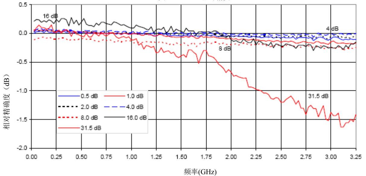
典型 AT4611 相对精度
