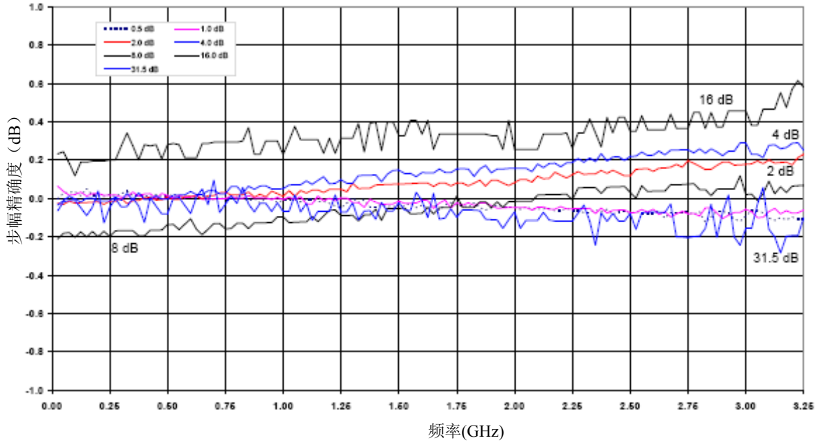
典型 AT4611 步幅精度
