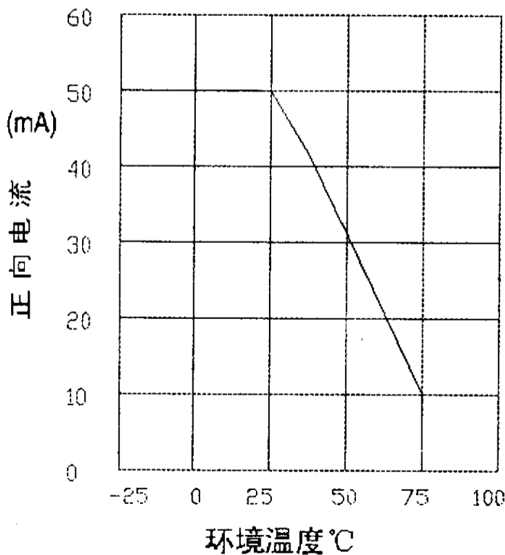
附图1. 正向电流与环境温度曲线图
