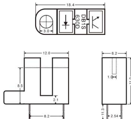
图.6 外形尺寸图 (单位: 毫米 ±0.1)
