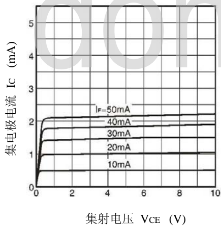
图.3 集电极电流与集射电压
