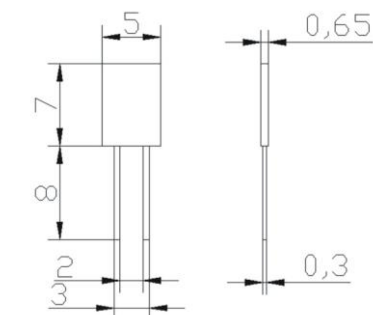
外形尺寸 (单位: mm)
