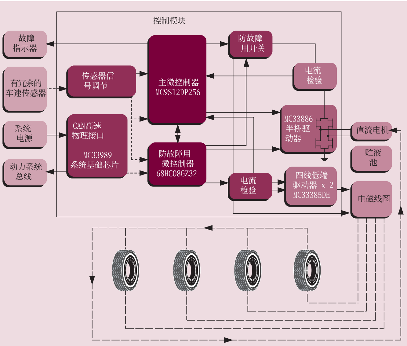
图 1. 防抱死制动系统控制模块
