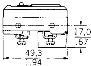
A28 6-32NC×.218”螺钉 可连接粗达 12 号线
