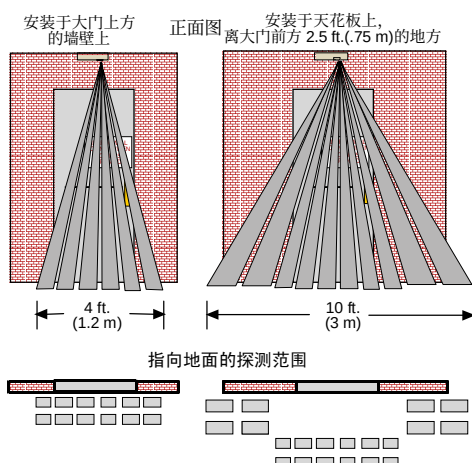
侧视图
