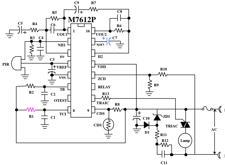
M7612 TCI PIN 外加電阻、電容與 Delay 時間的關
