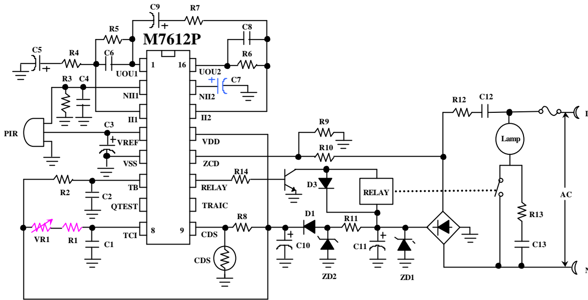
M7612 TCI PIN 外加电阻、电容与 Delay 时间的关
