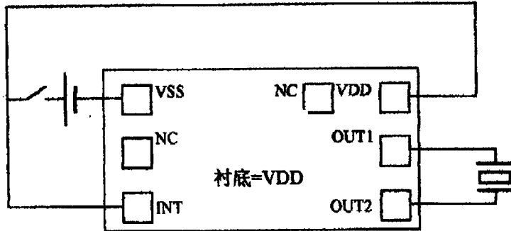
1: 连响模式应用电路图
