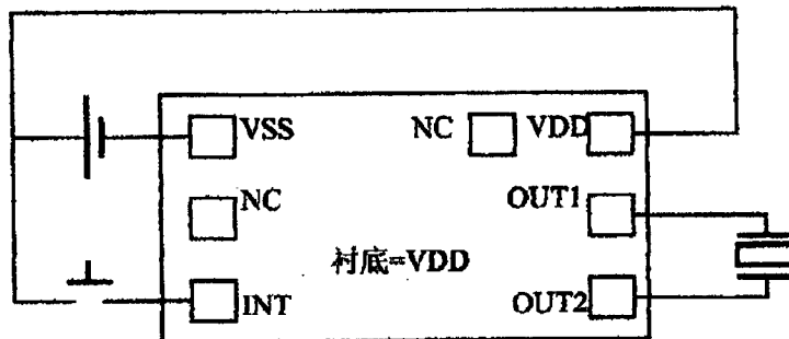
2: 触发模式应用电路图
